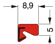
Überschlagdichtung 2nd sash-seal
