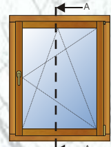
Überschlagdichtung 2nd sash-seal
