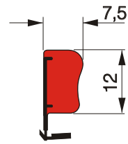
Überschlagdichtung 2nd sash-seal
