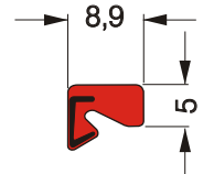
Überschlagdichtung 2nd sash-seal
