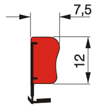
Überschlagdichtung 2nd sash-seal
