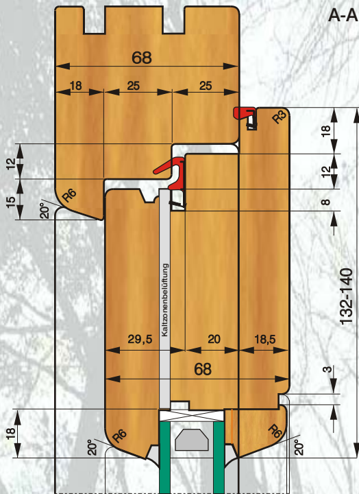
A-A
